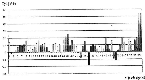
Hình 2. Biểu đồ thể hiện sự thay đổi diện tích tại các mặt cắt giai đoạn 1993-1996
